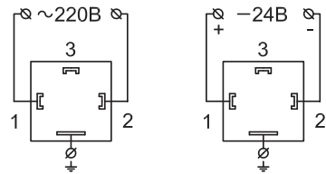
Схема подключения катушки
